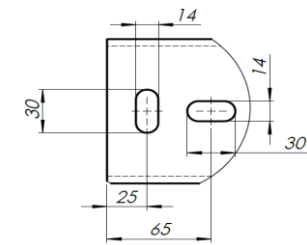
Montage des Trägerprofil am Transportförderer
